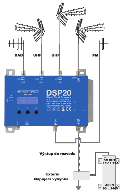
Dálkové napájení DSP20 přes výstupní konektor
